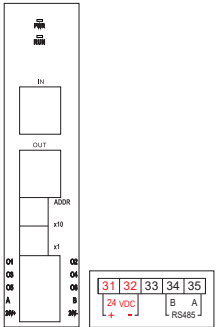
D92D 外形及接线图 (V2.0 )
