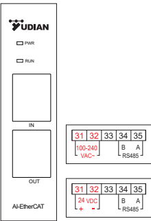
D71 外形及接线图
